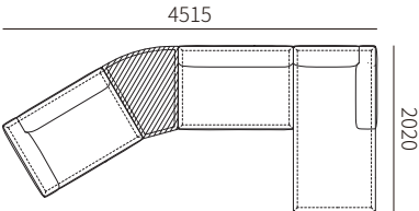
HW03A-1R + HW03E-2 + HW03B-1 + HW03C-2L 4515*2020*660MM 177.8*79.5*26.0"
